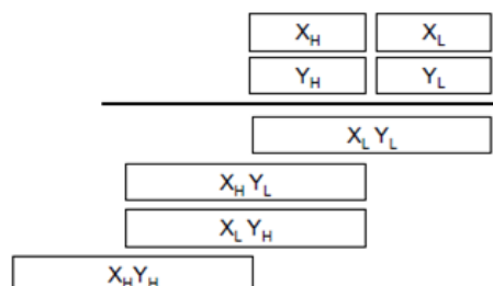
Fig.6: 8x8 Multiplier using 4x4 Multiplier
